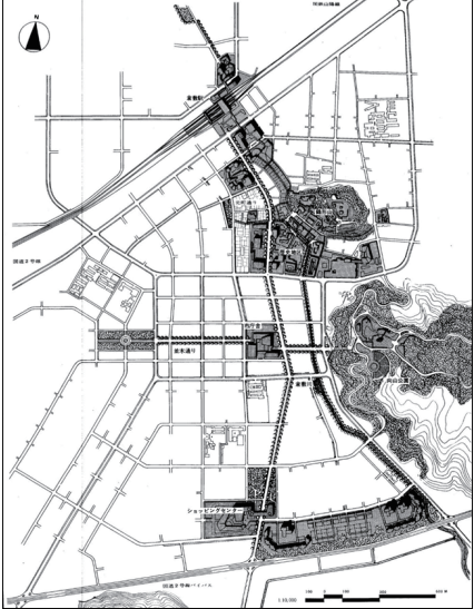
【1967(昭和 42)年】倉敷市中心部地区設計案 出典：東京大学都市工学科編「倉敷市の将来像に関する懇談会報告」倉敷市の将来像に関する懇談会、1967
